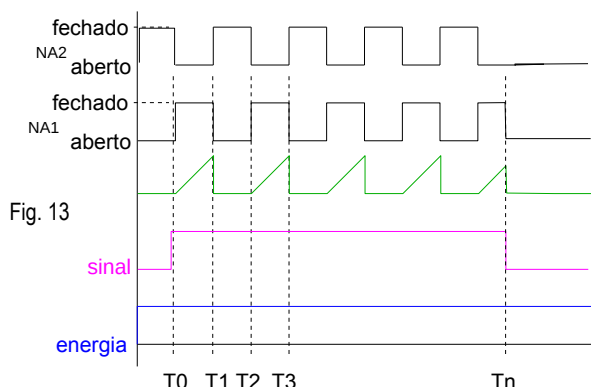
Graf. 4 Temporizador Cíclico Complementar. Config.E = 8 (Temporizador Cíclico Complementar) Config.t = 4 (Timer Cíclico) + 16 (Partida por sinal externo nível alto /baixo).
